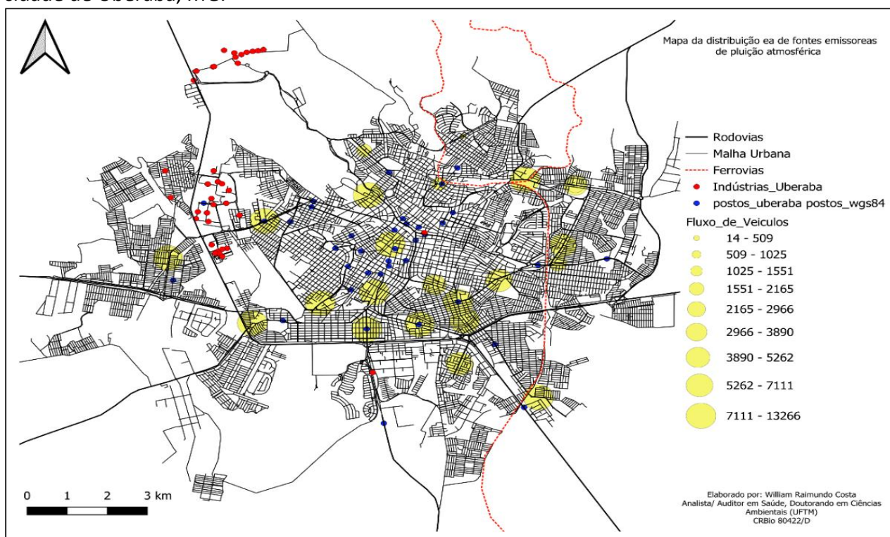
Figura 02 – Mapa preliminar da distribuição de fontes emissoras de poluentes atmosféricos da cidade de Uberaba, MG.
